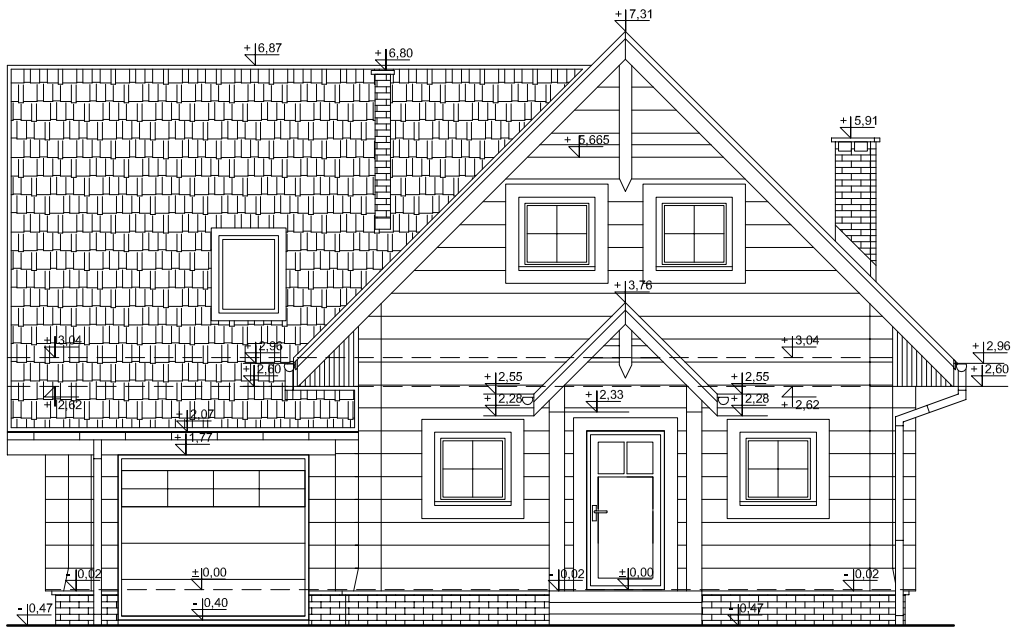
ELEWACJA FRONTOWA
